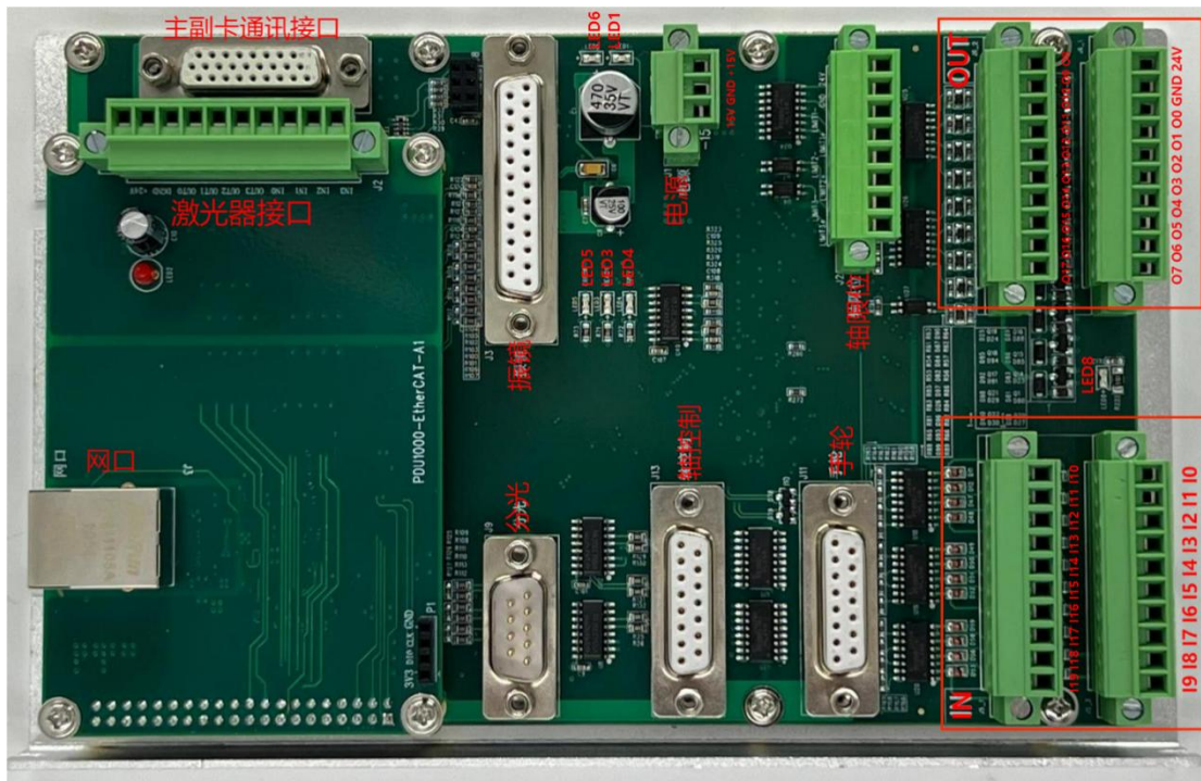
PCIE 端子板
