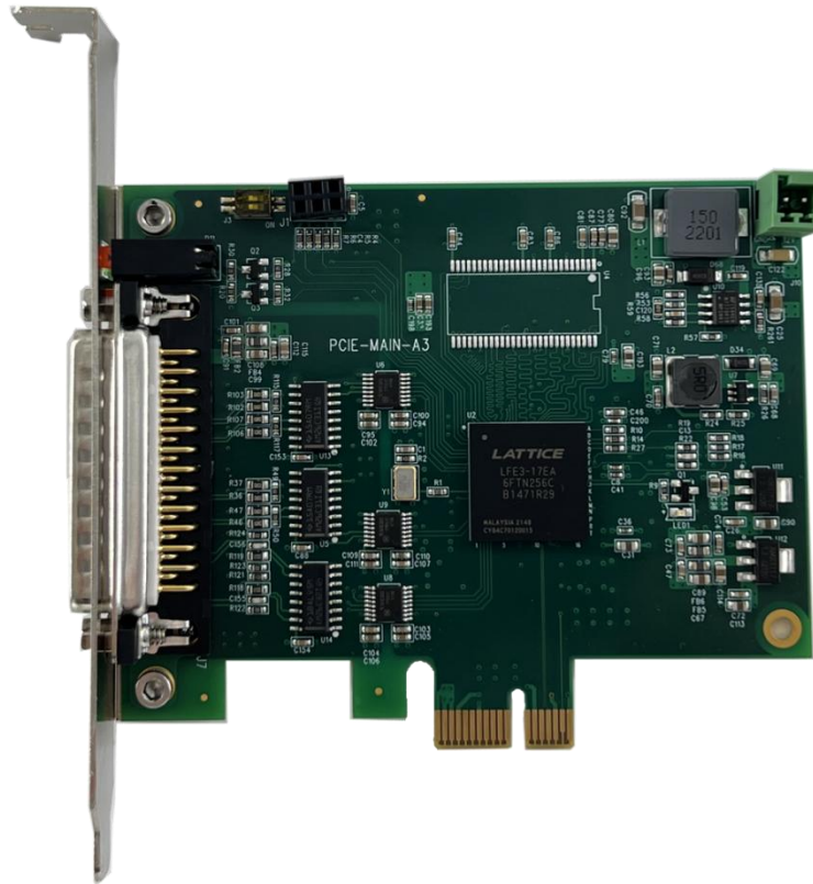
PCIE 主卡
