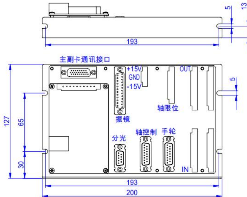
PCIE 端子板
