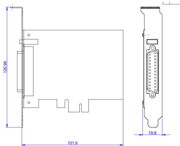
PCIE 主卡
